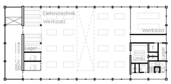
HWK Hauptgebäude 3 - OG2 | M1:500
