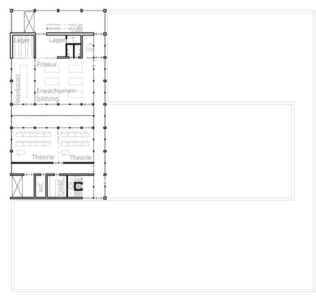
HWK Hauptgebäude 2 - OG4 | M1:500
