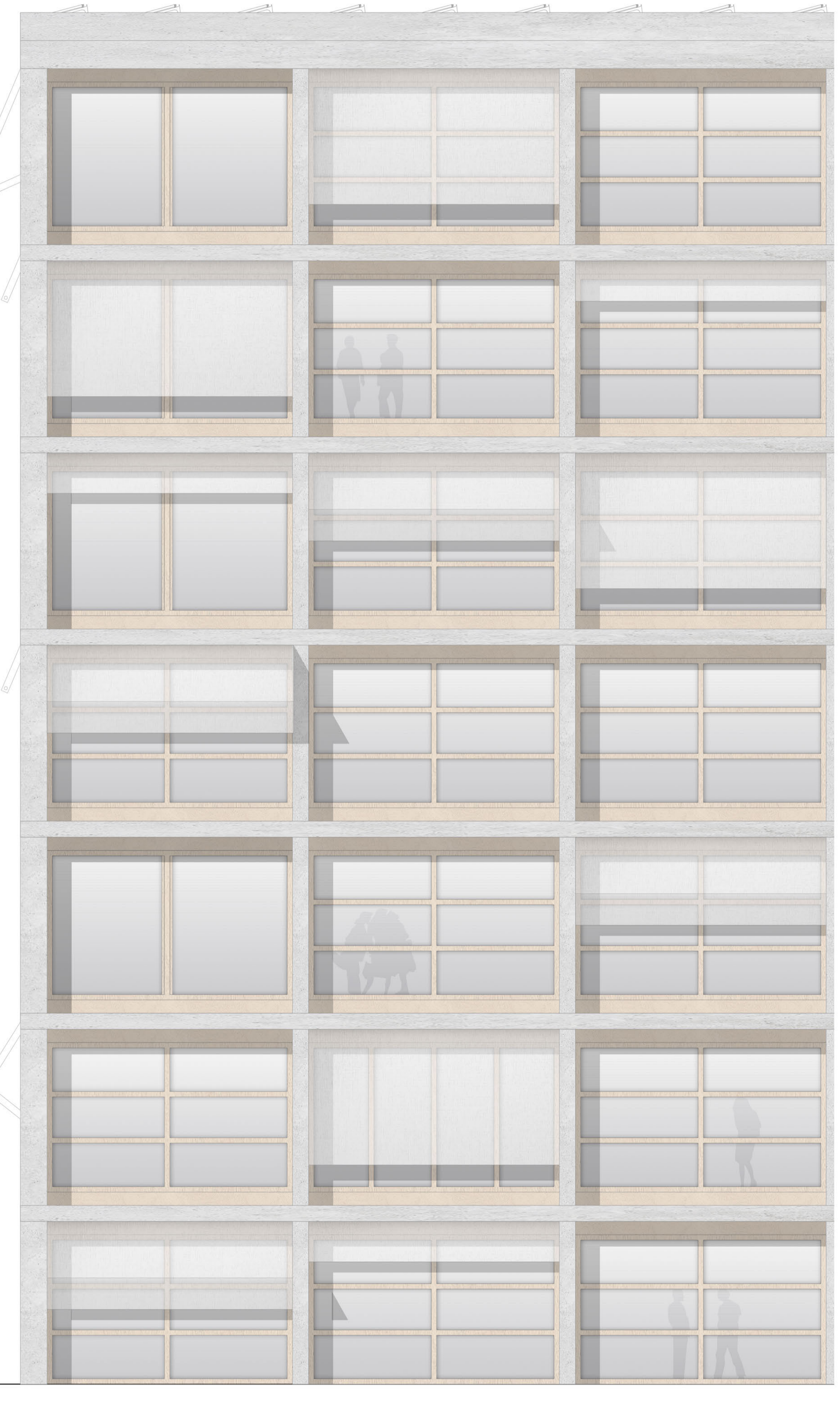
Konstruktive Vertiefung - Ansicht | M1:50
