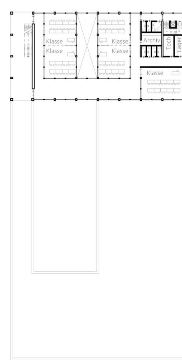
PHS - OG4 | M1:500
