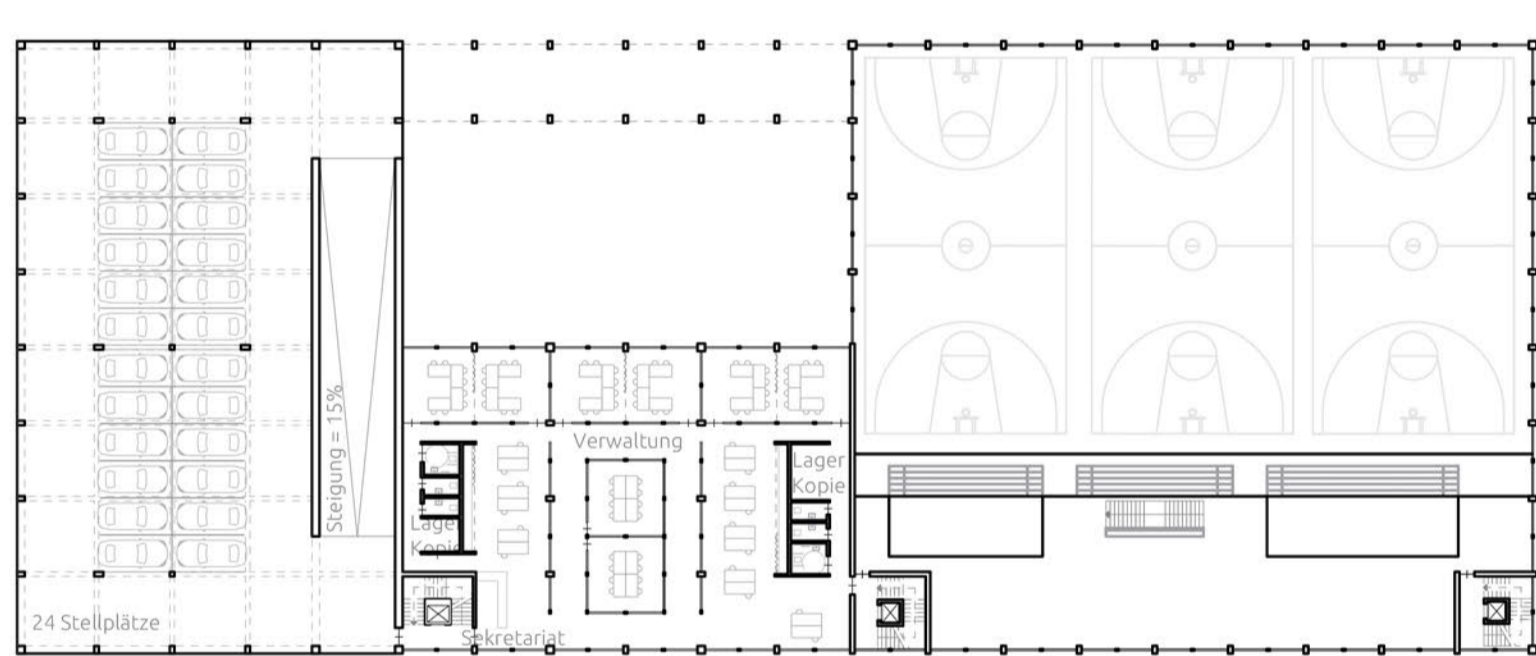
Parkhaus, Internat, Verwaltung - OG2 | M1:500
