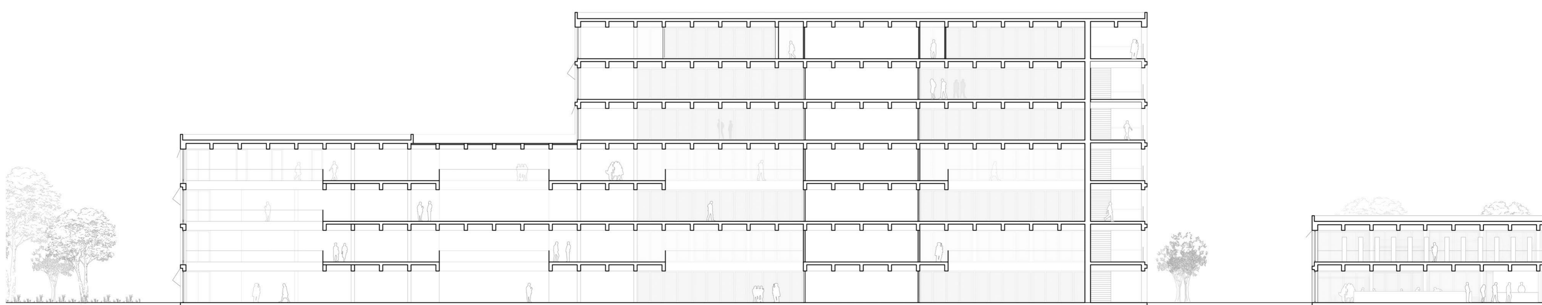
Schnitt B-B | M1:200
