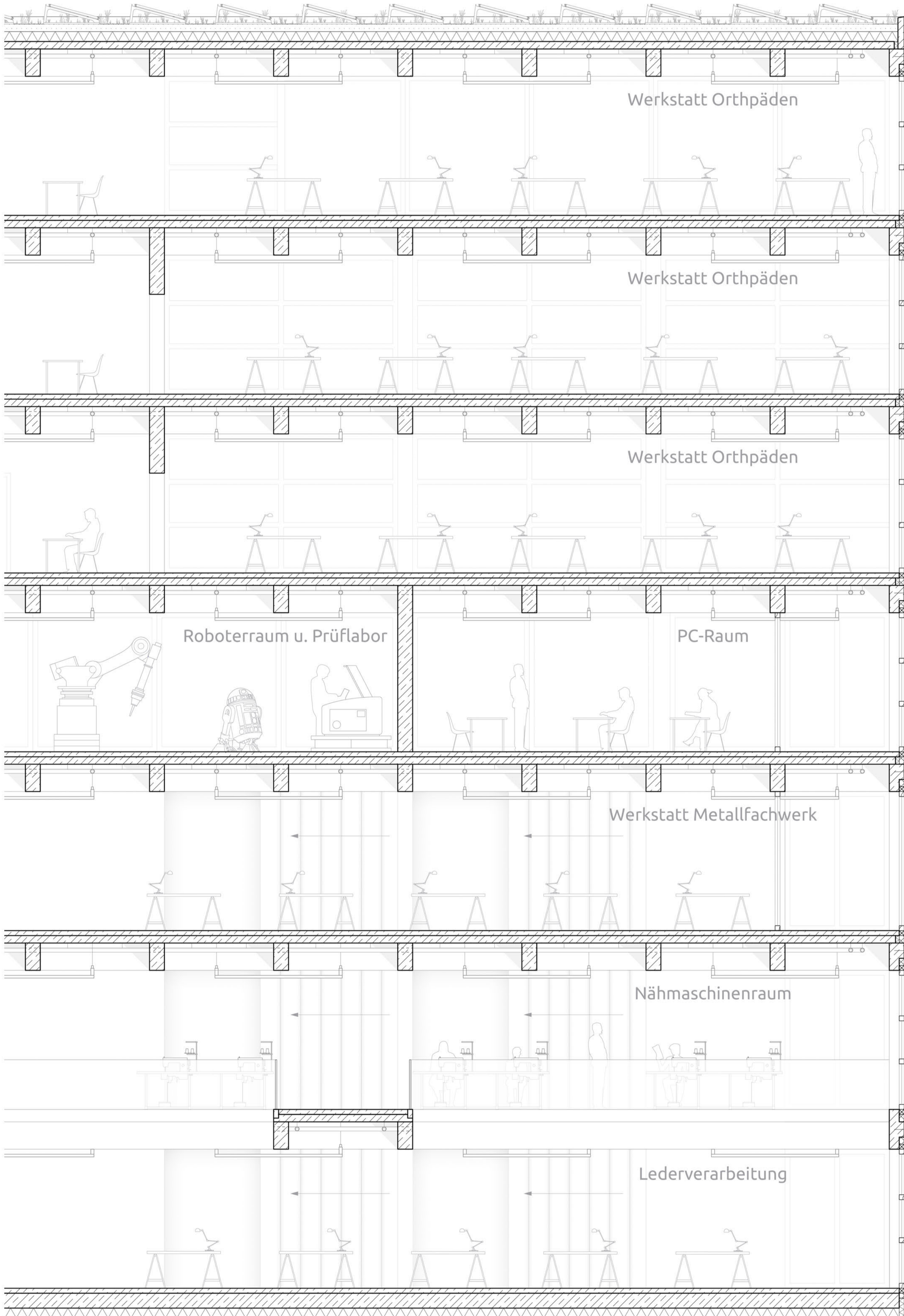
Konstruktive Vertiefung - Schnitt | M1:50
