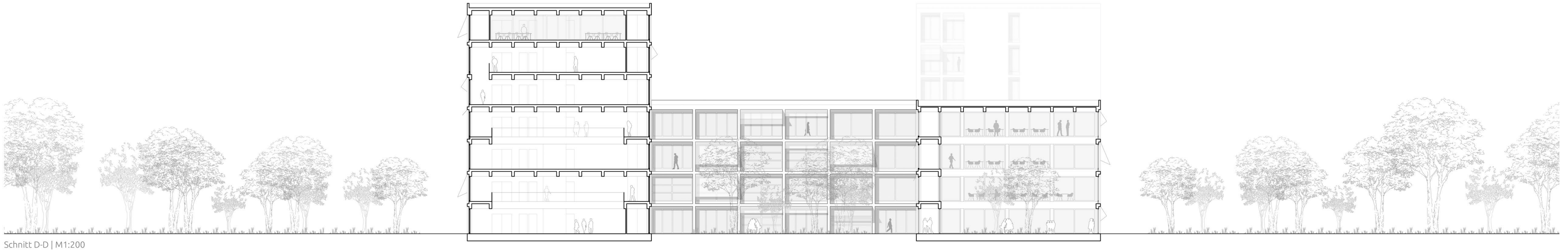
Schnitt D-D | M1:200
