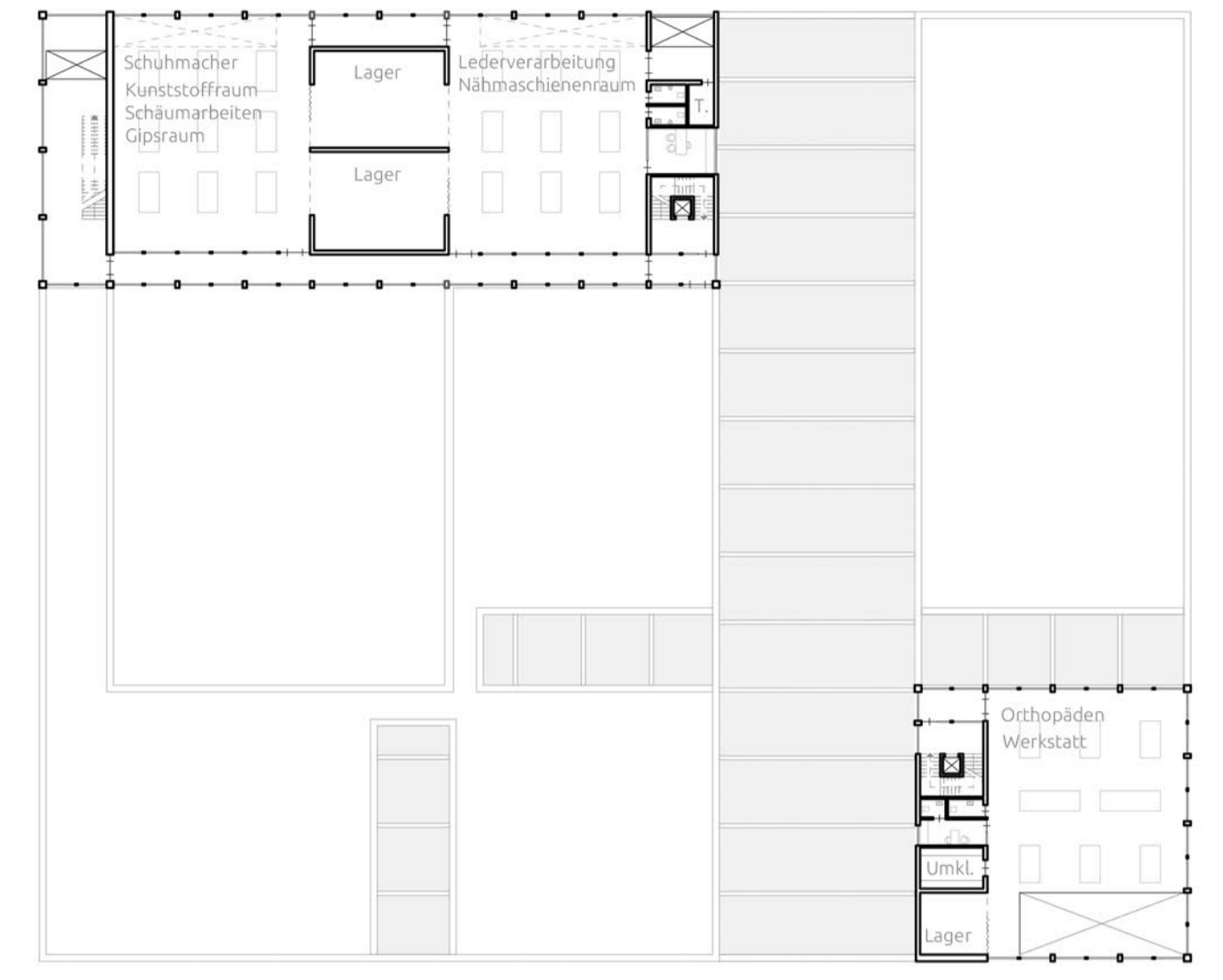
HWK Hauptgebäude 1 - OG4 | M1:500
