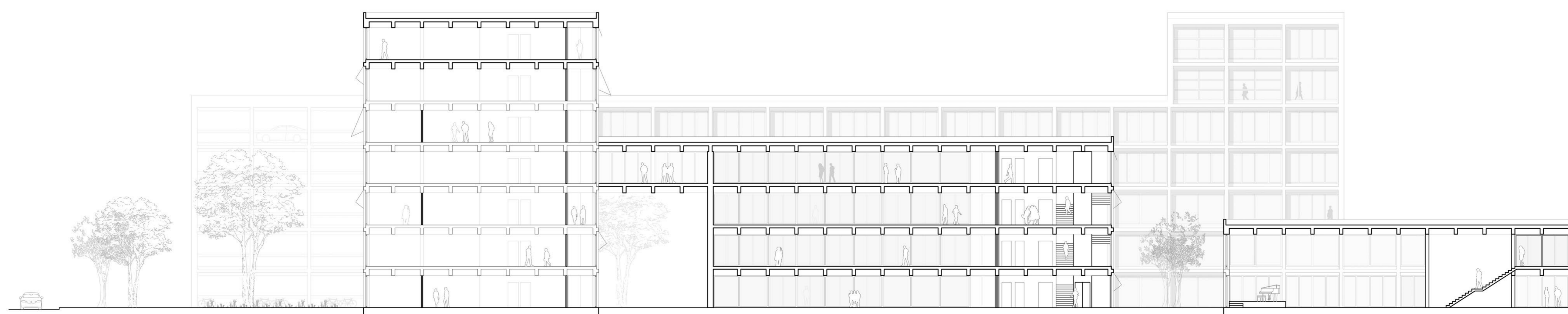
Schnitt A-A | M1:200
