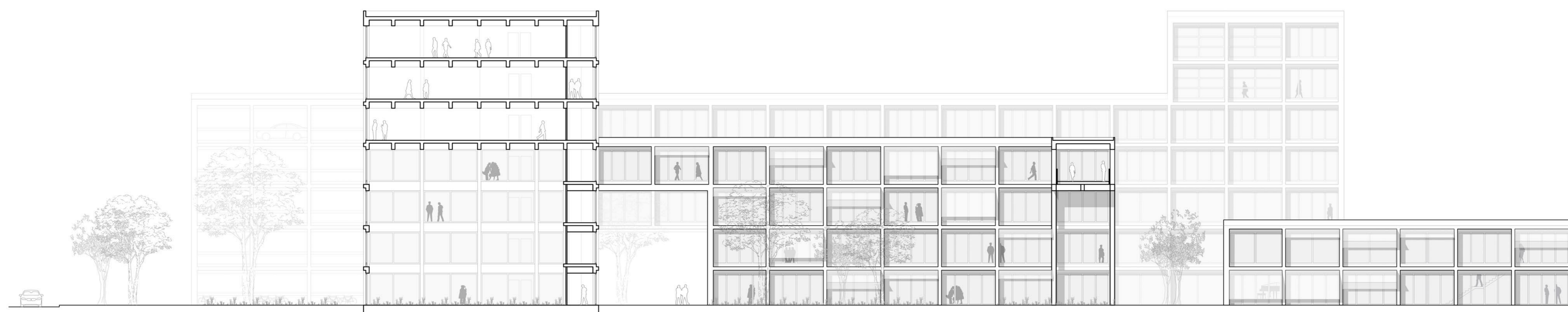
Ansicht Süd / Schnittansicht F-F | M1:200
