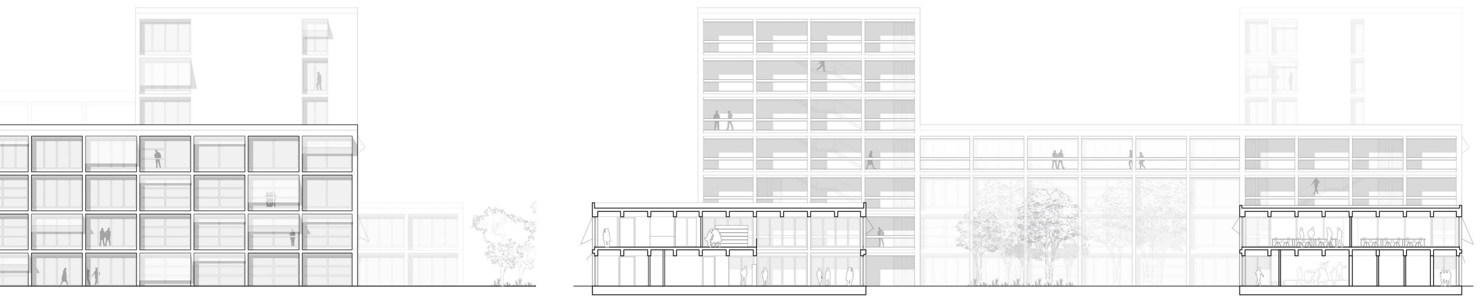
Schnittansicht West / Schnitt E-E | M1:200
