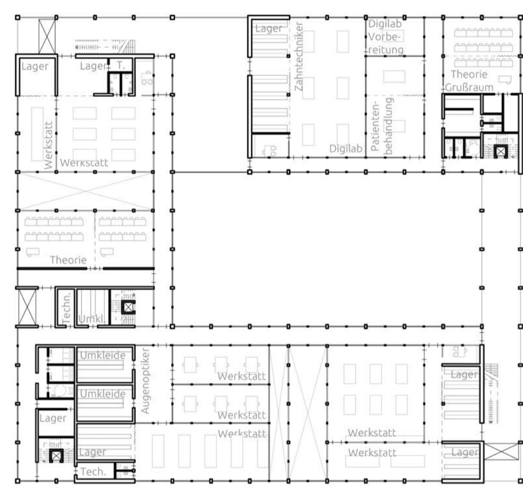
HWK Hauptgebäude 2 - OG3 | M1:500
