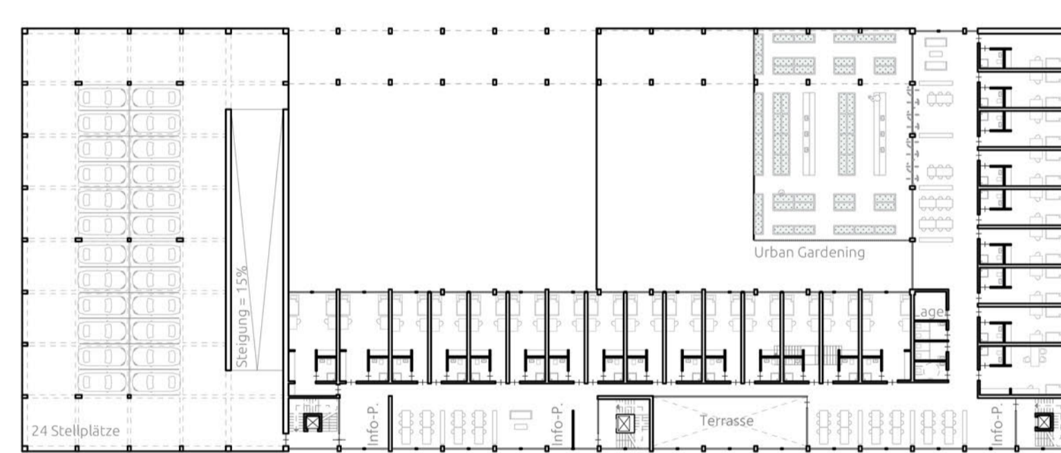
Parkhaus, Internat, Verwaltung - OG3 | M1:500
