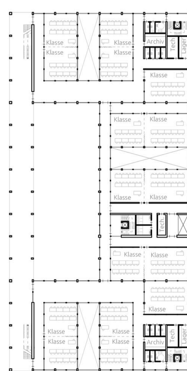
PHS - OG3 | M1:500
