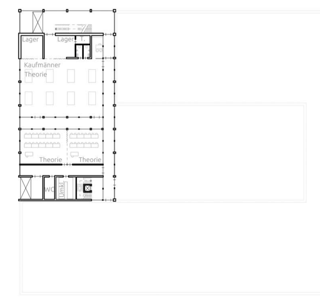
HWK Hauptgebäude 2 - OG6 | M1:500
