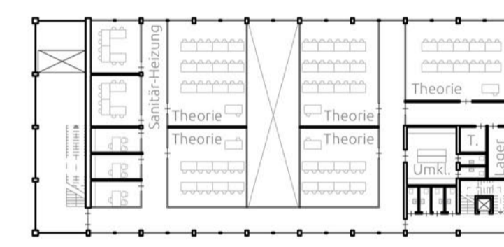
HWK Hauptgebäude 3 - OG7 | M1:500
