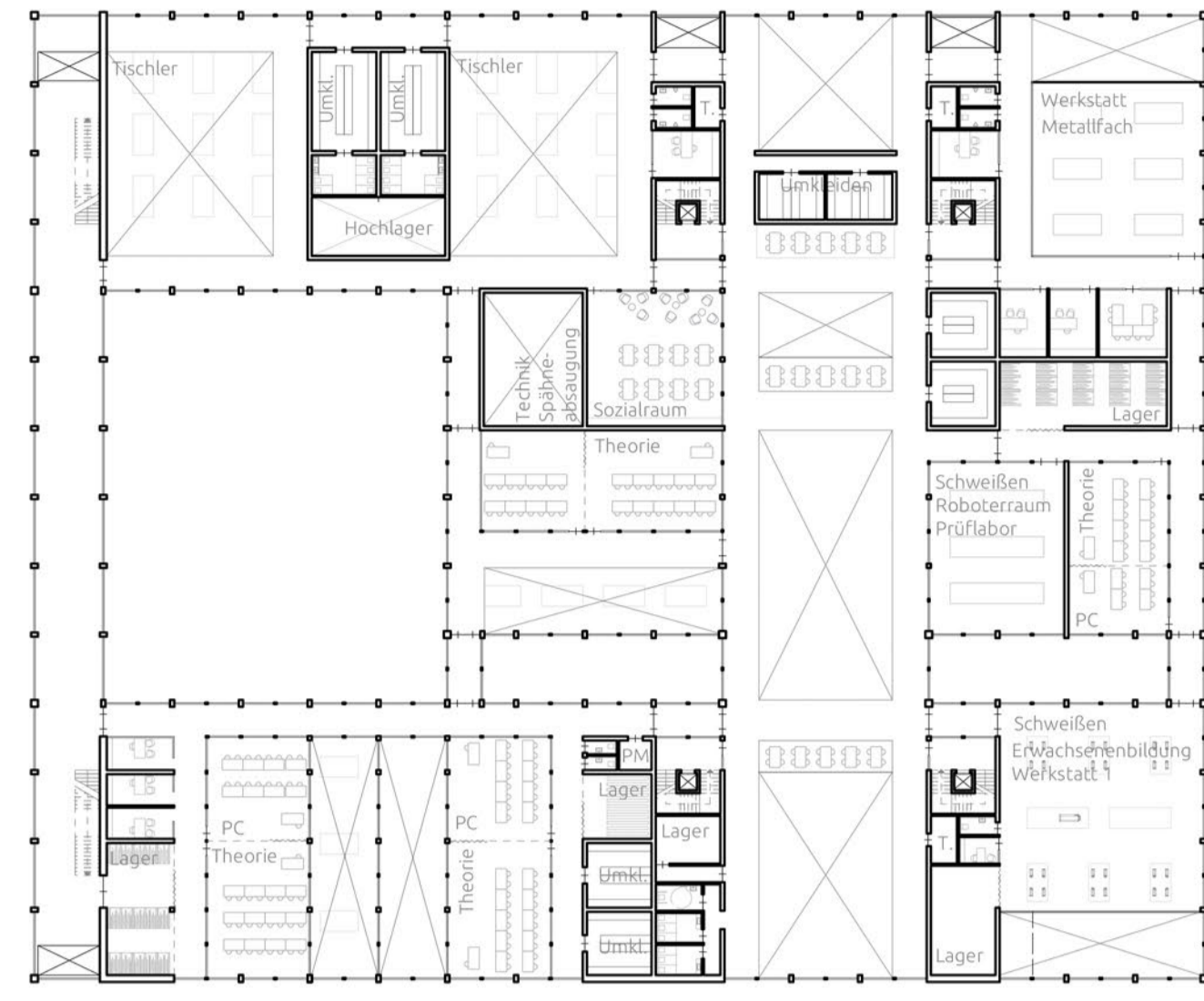
HWK Hauptgebäude 1 - OG3 | M1:500
