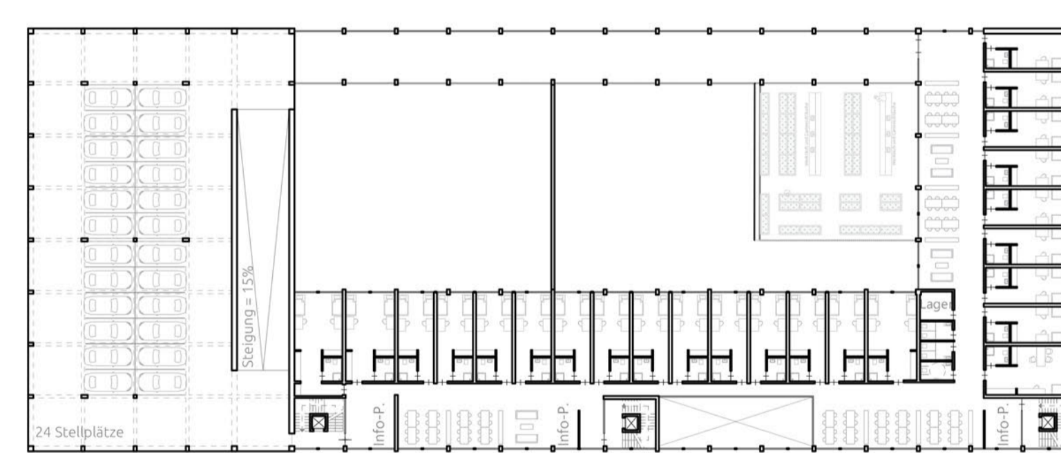
Parkhaus, Internat, Verwaltung - OG4 | M1:500
