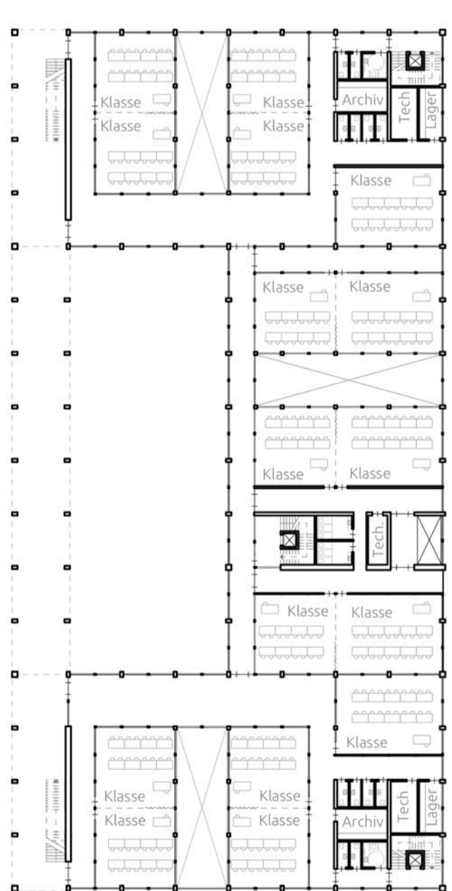
PHS - OG2 | M1:500
