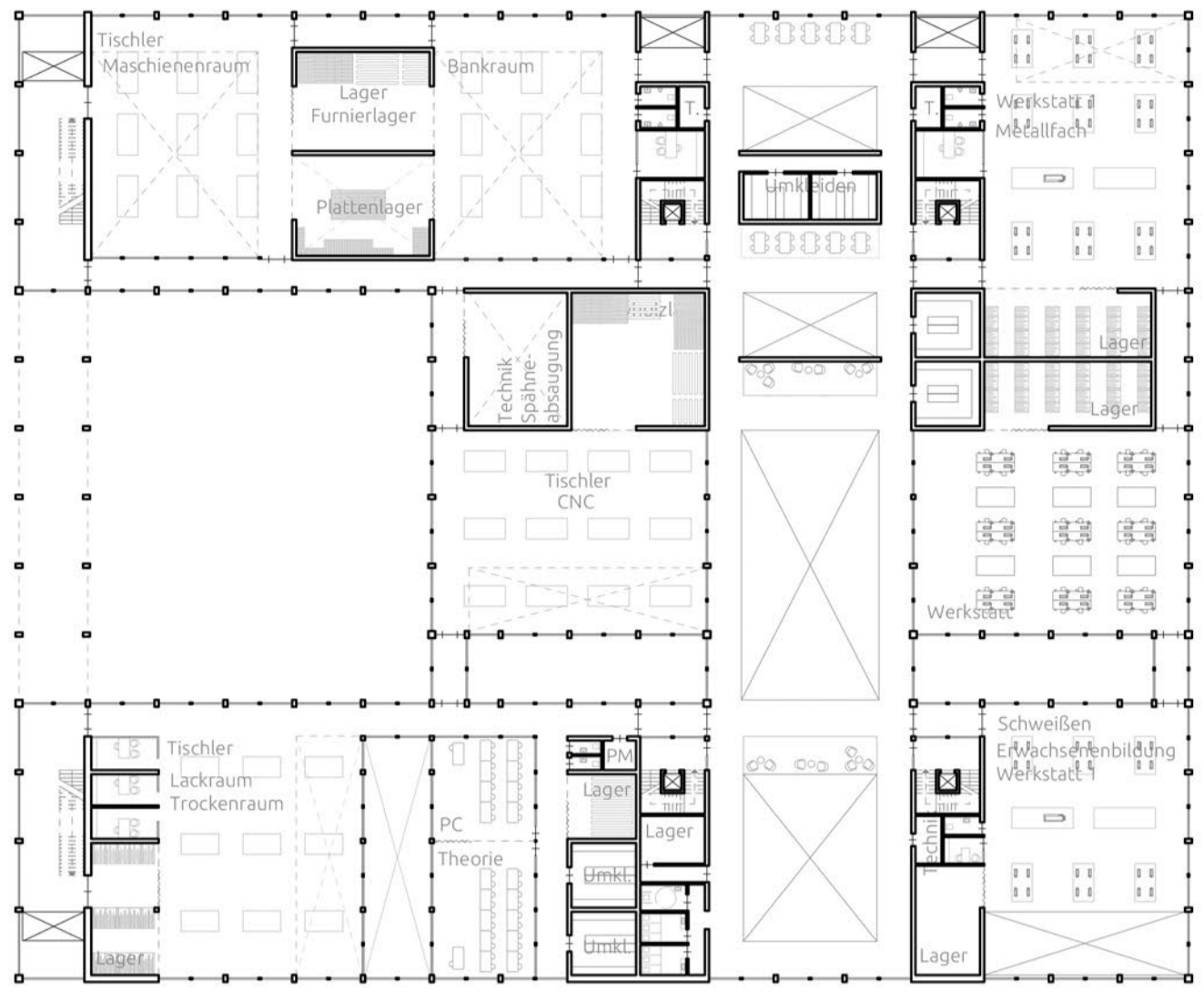
HWK Hauptgebäude 1 - OG2 | M1:500
