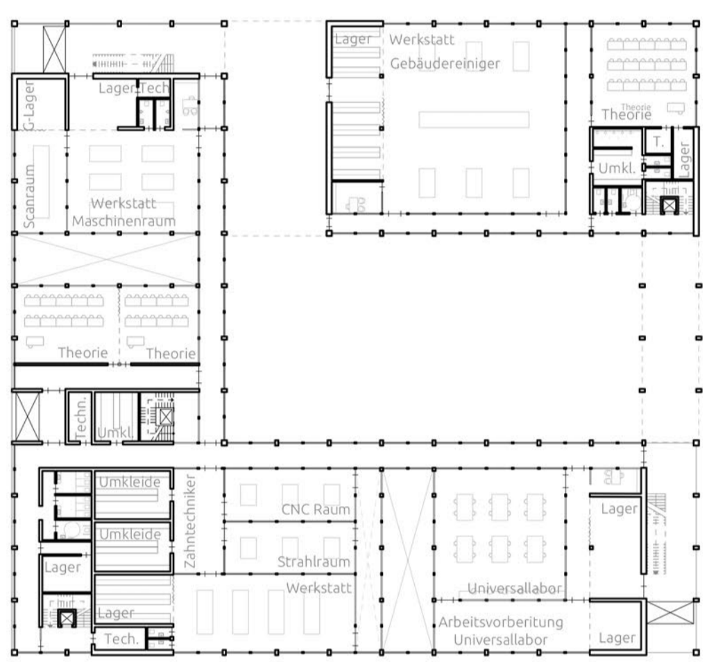
HWK Hauptgebäude 2 - OG2 | M1:500
