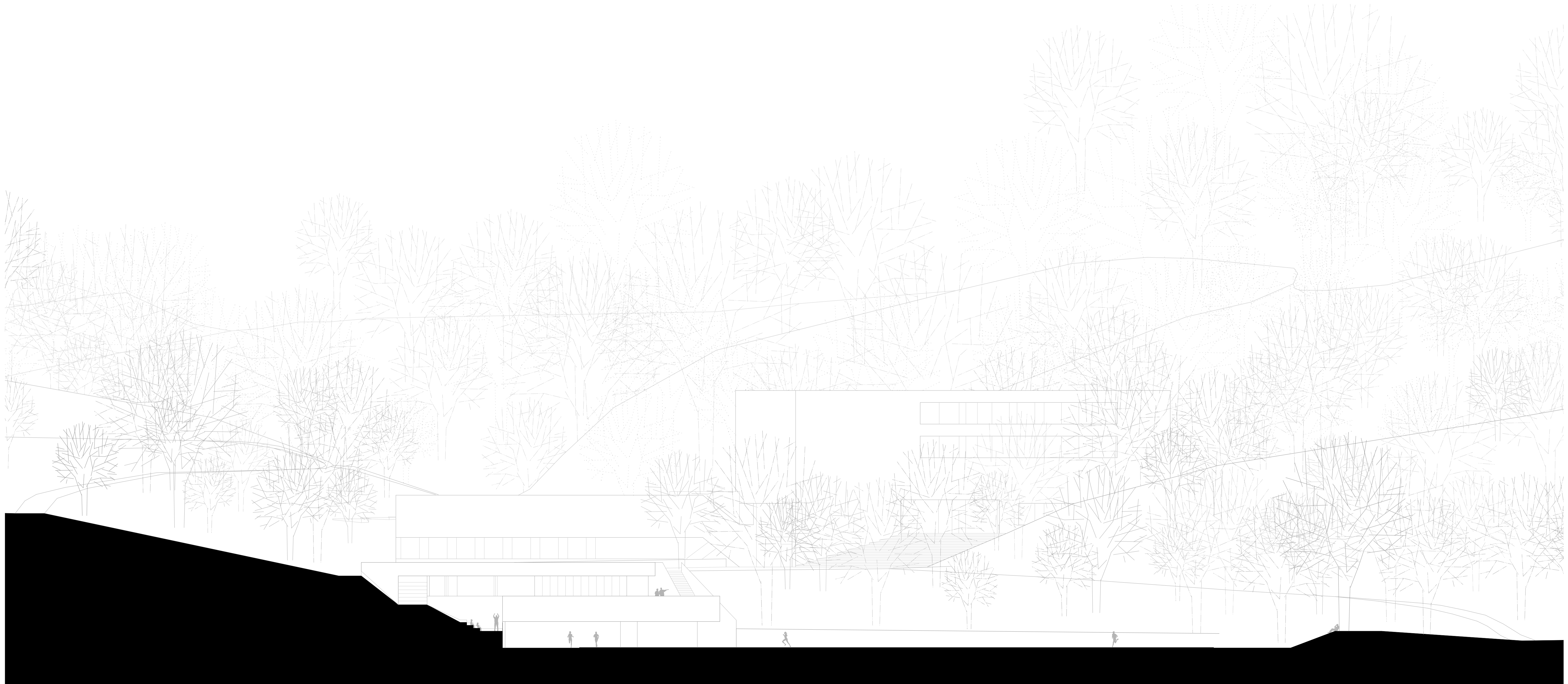
Schnitt_Stadion quer_Ansicht Sportzentrum_M 1.200
