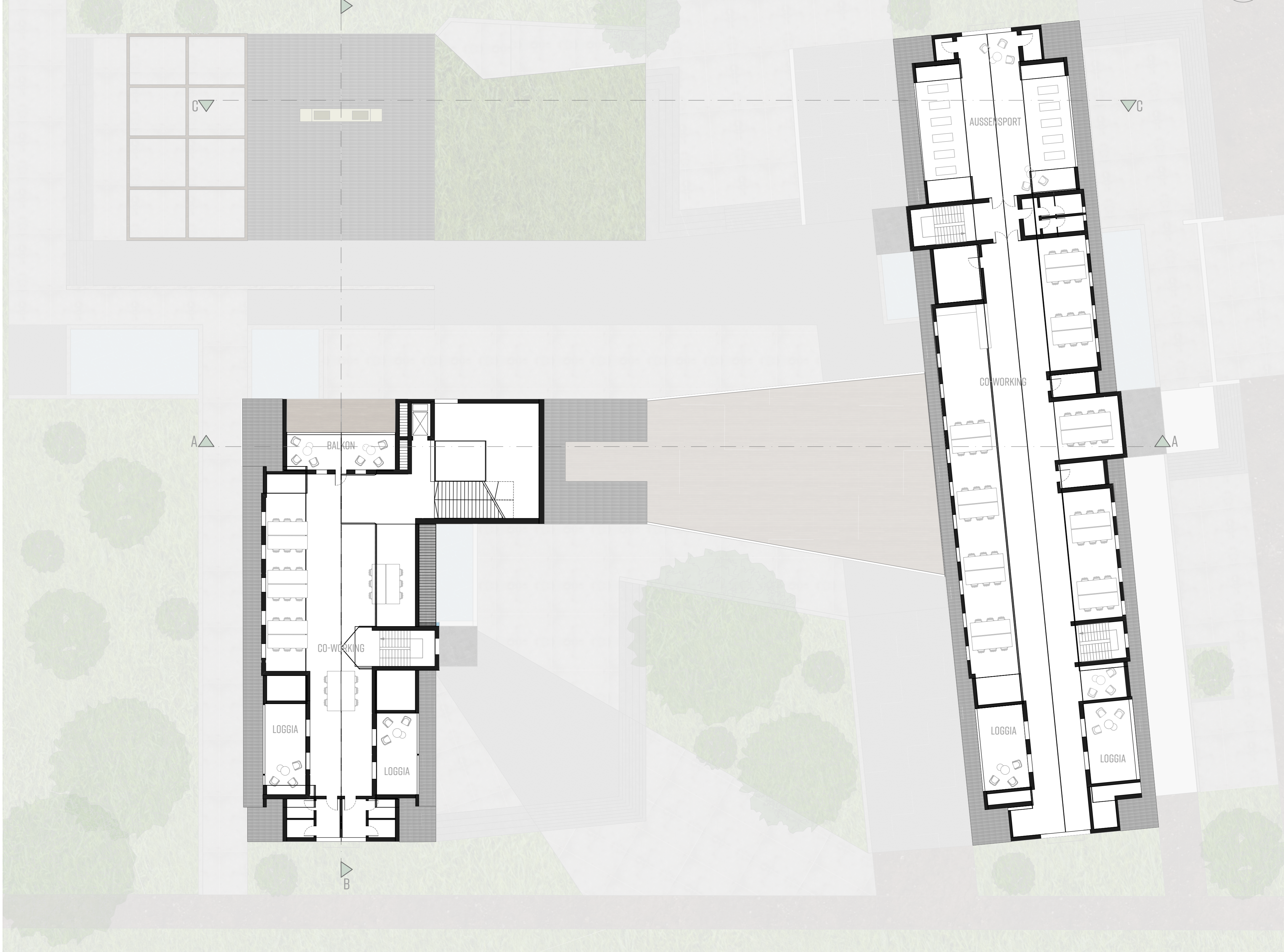
GRUNDRISS DACHGESCHOSS M 1:200
