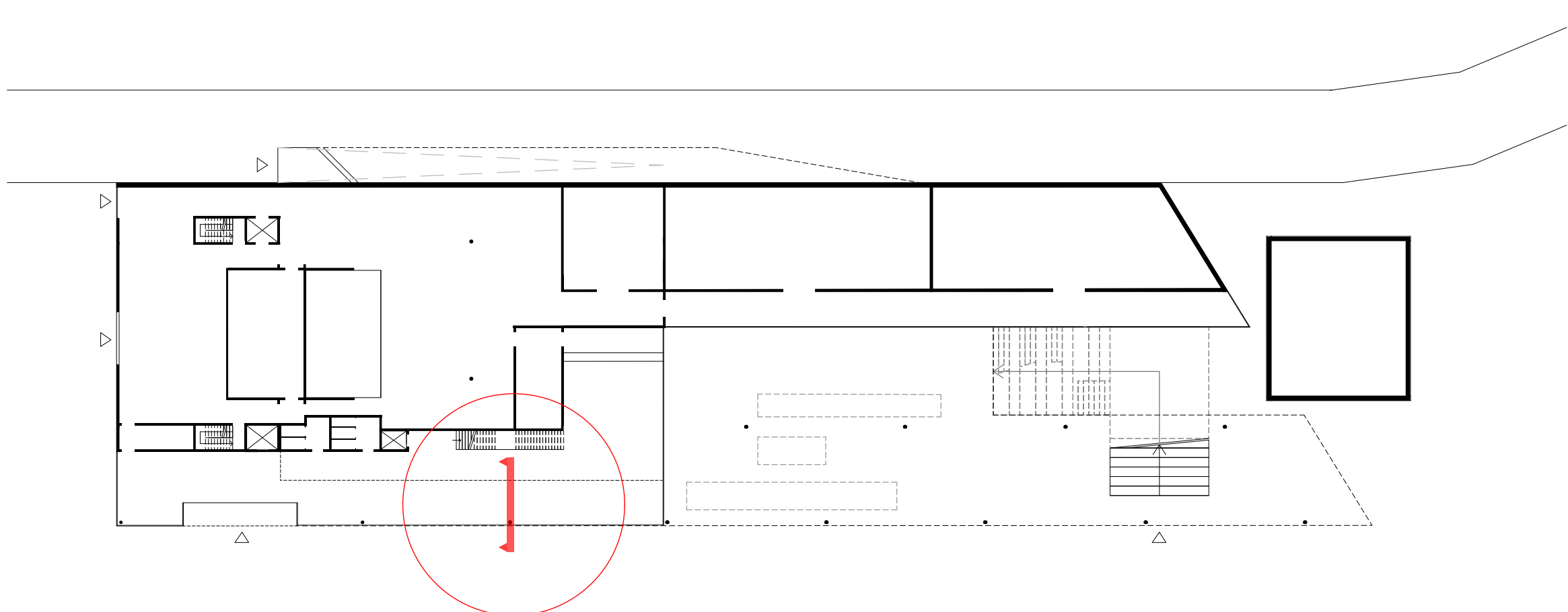
Grundriss Schnittpunkt
