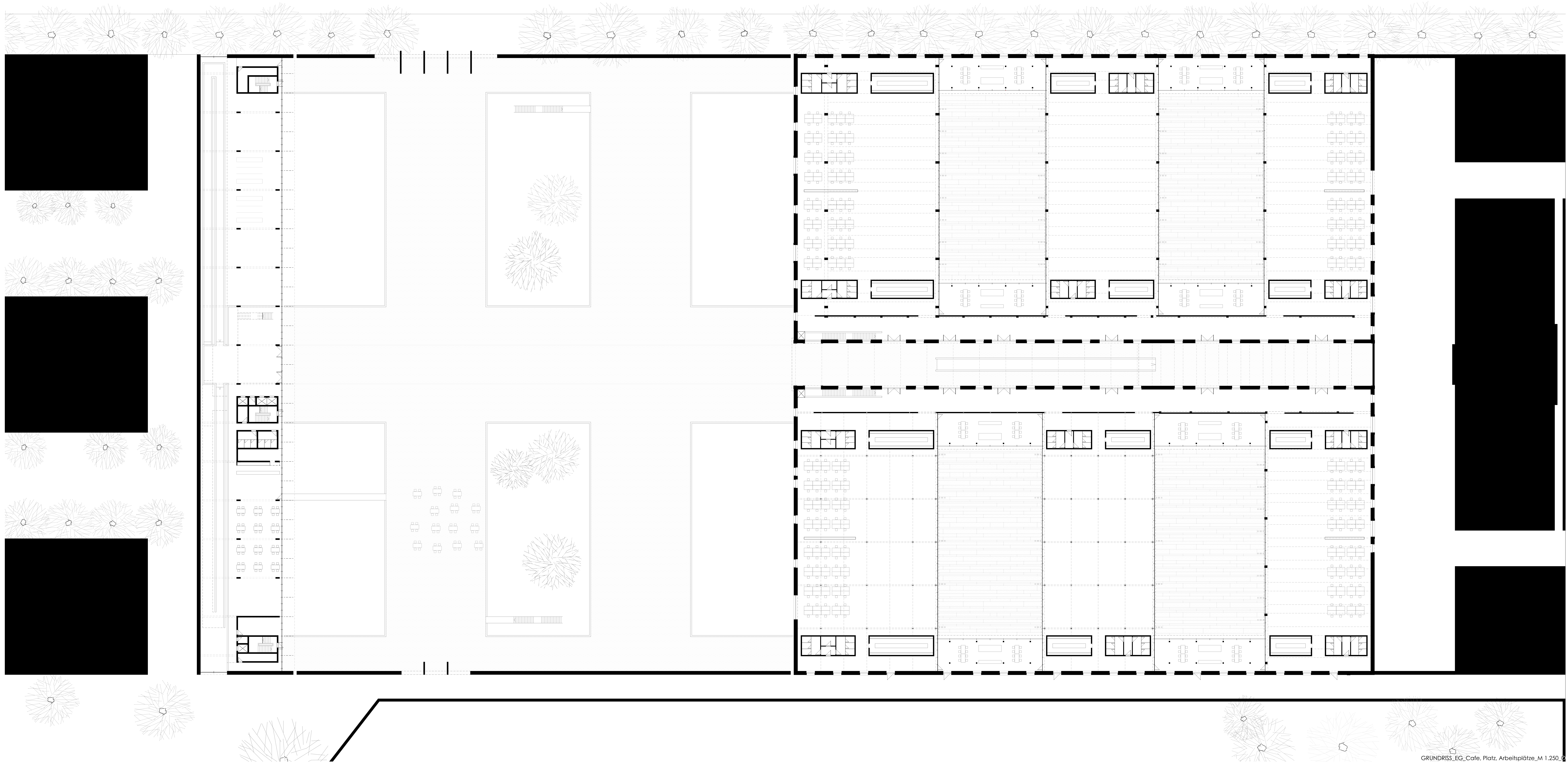
GRUNDRISS_EG_Cafe, Platz, Arbeitsplätze_M 1:250
