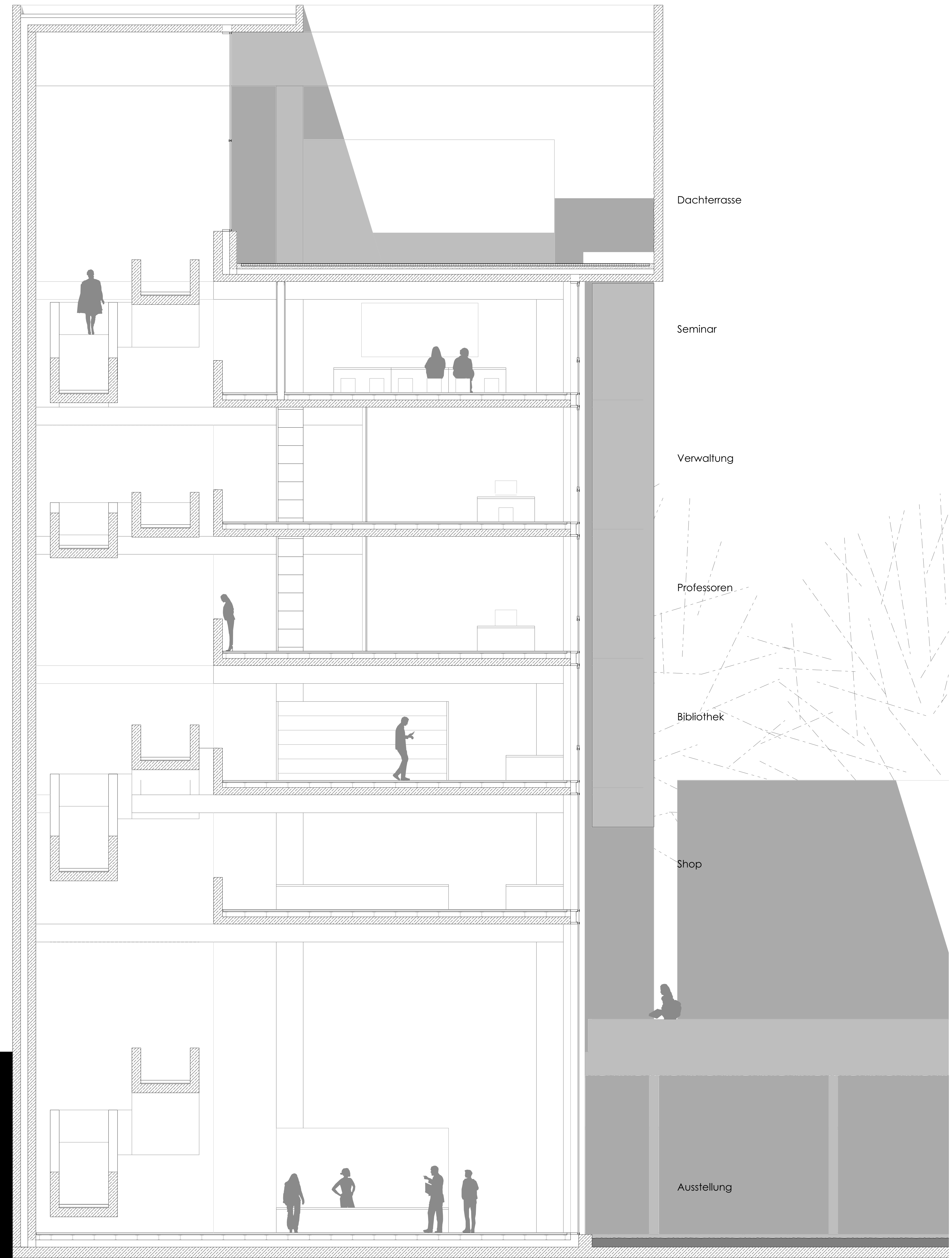
SCHNITT Riegel_M 1:50
