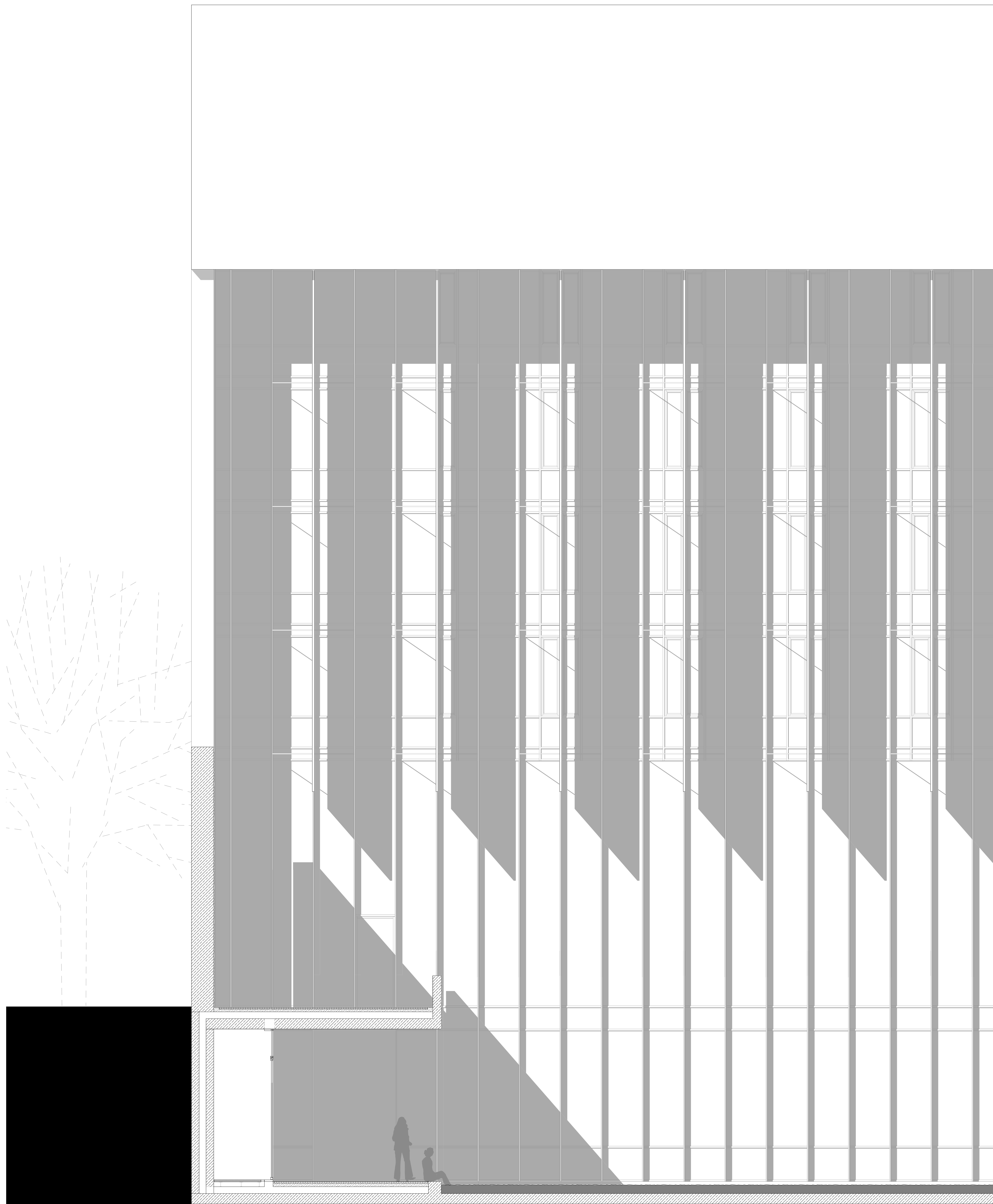
SCHNITT Riegel Fassade_M 1:50
