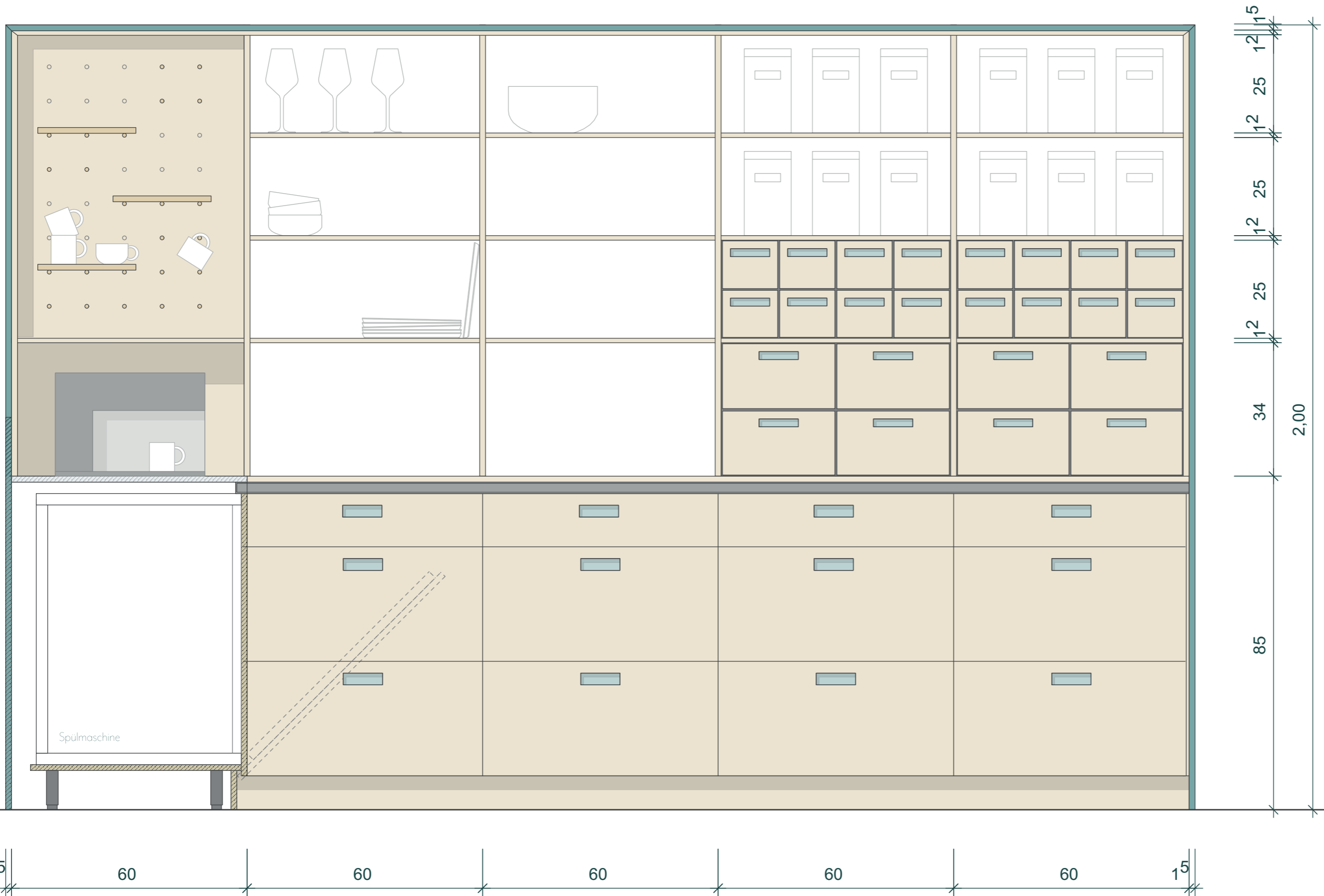
Längsschnitt M 1:10
